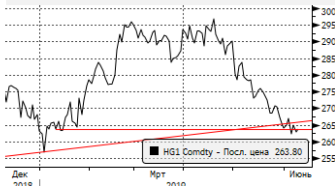
Медь: тест уровней поддержки
