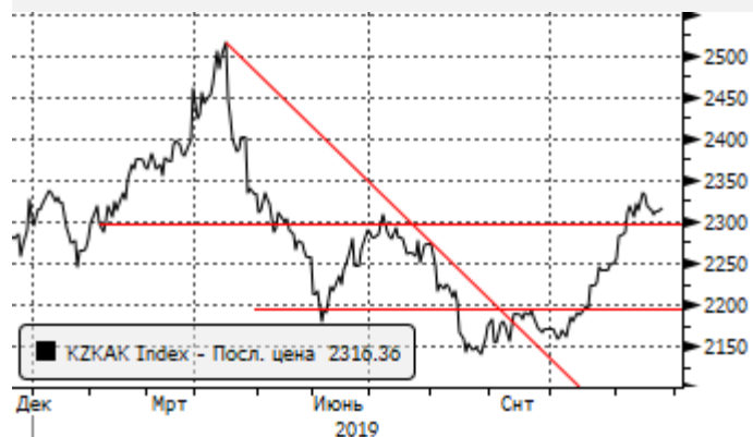
KASE: отыграна нисходящая дивергенция
